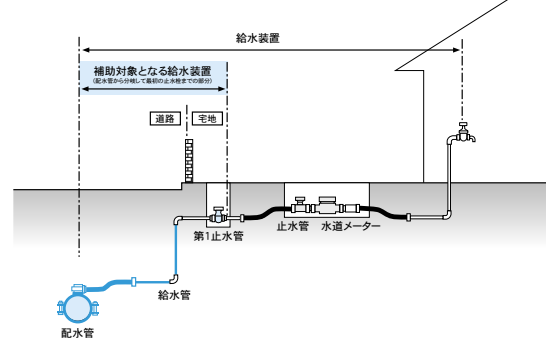
■図1 給水装置の設置例
