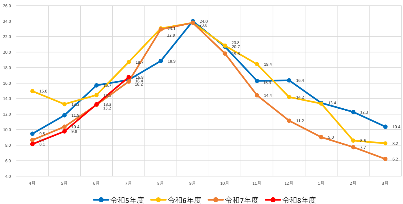
広田湾漁場水質調査 海水温各年度比較（要谷沖） 水深10m地点
