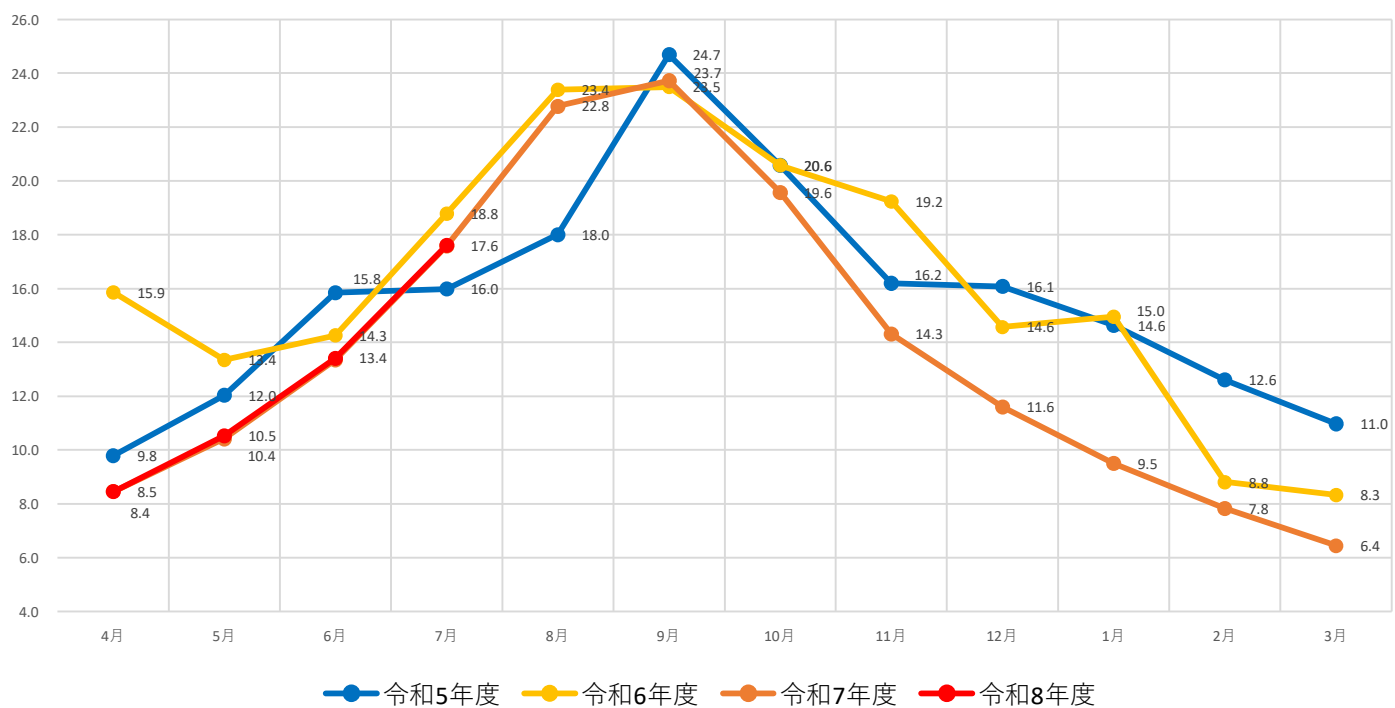
広田湾漁場水質調査 海水温各年度比較（泊沖） 水深10m地点
