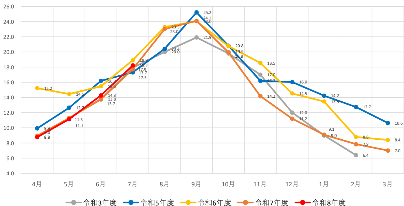
広田湾漁場水質調査 海水温各年度比較（福伏沖） 水深5m地点
