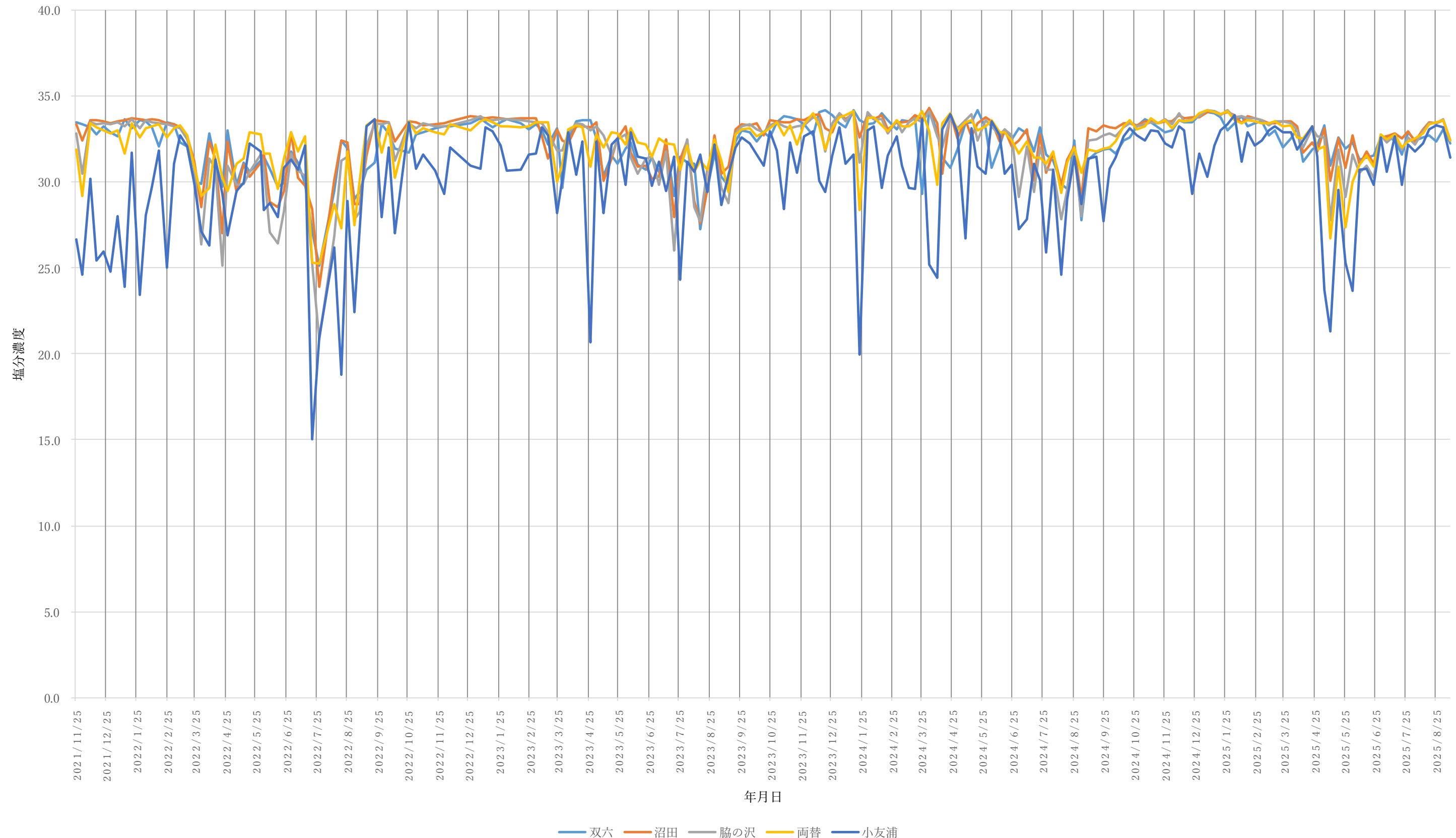
広田湾奥漁港内塩分濃度（PSU）
