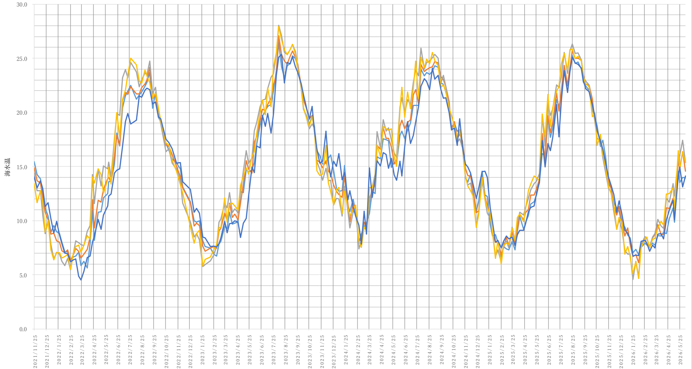
広田湾奥漁港内海水温(°C)
