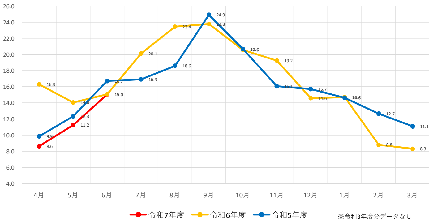
広田湾漁場水質調査 海水温各年度比較（泊沖）
