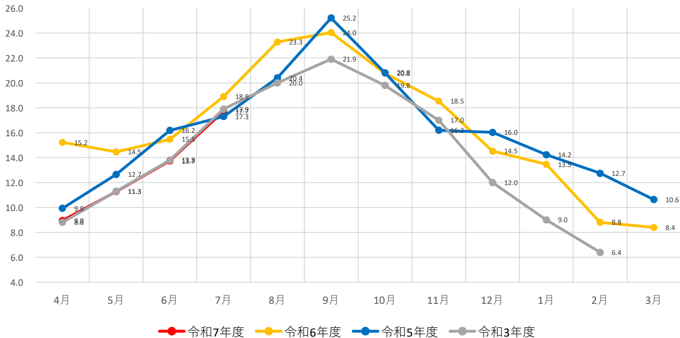
広田湾漁場水質調査 海水温各年度比較（福伏沖）
