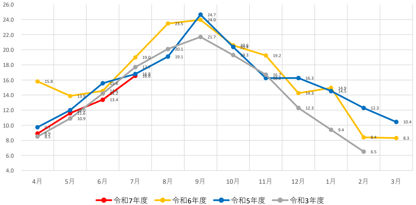
広田湾漁場水質調査 海水温各年度比較（大陽沖）
