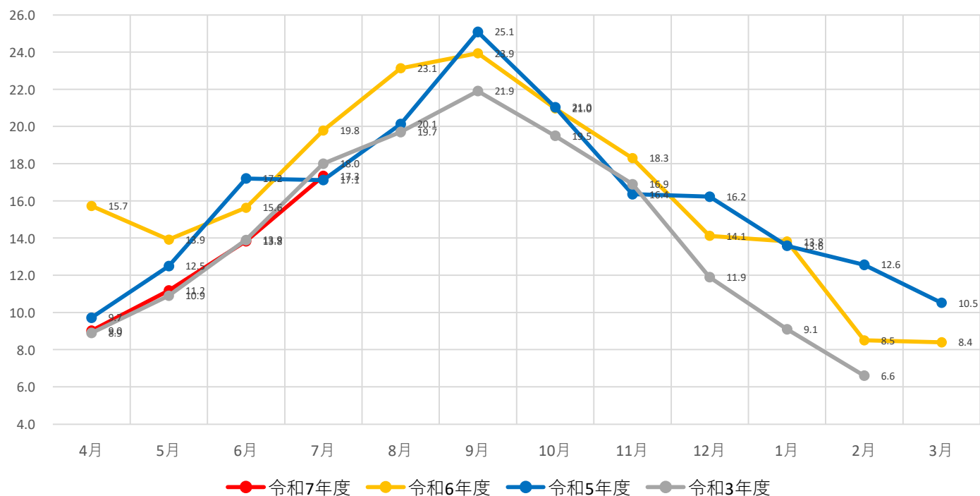
広田湾漁場水質調査 海水温各年度比較（高田沖）
