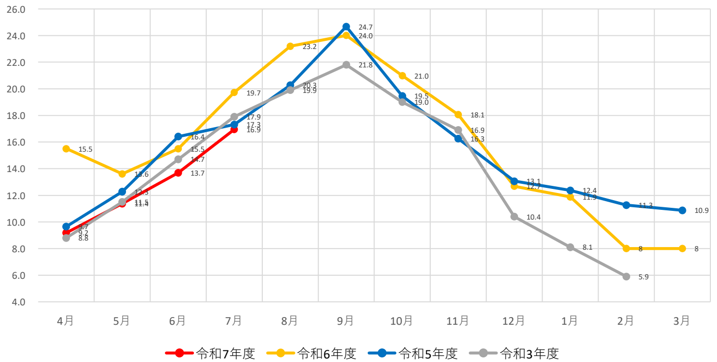
広田湾漁場水質調査 海水温各年度比較（小友浦沖）
