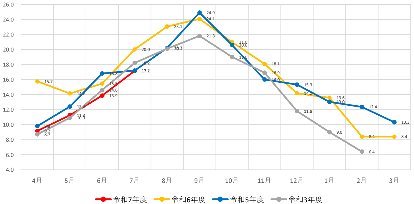
広田湾漁場水質調査 海水温各年度比較（脇之沢沖）
