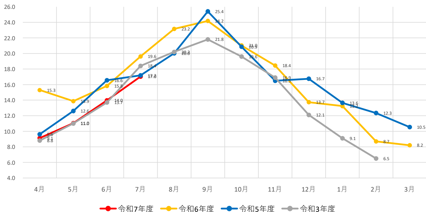
広田湾漁場水質調査 海水温各年度比較（長部沖）
