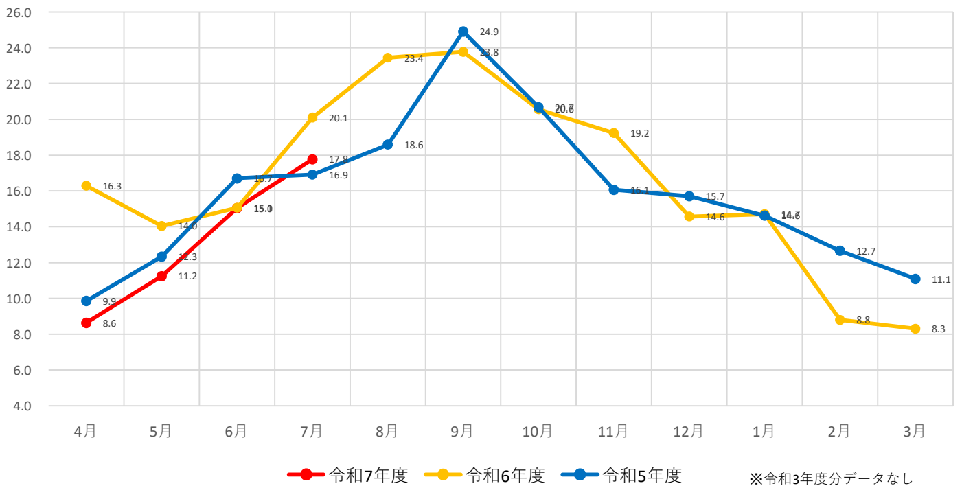
広田湾漁場水質調査 海水温各年度比較（泊沖）
