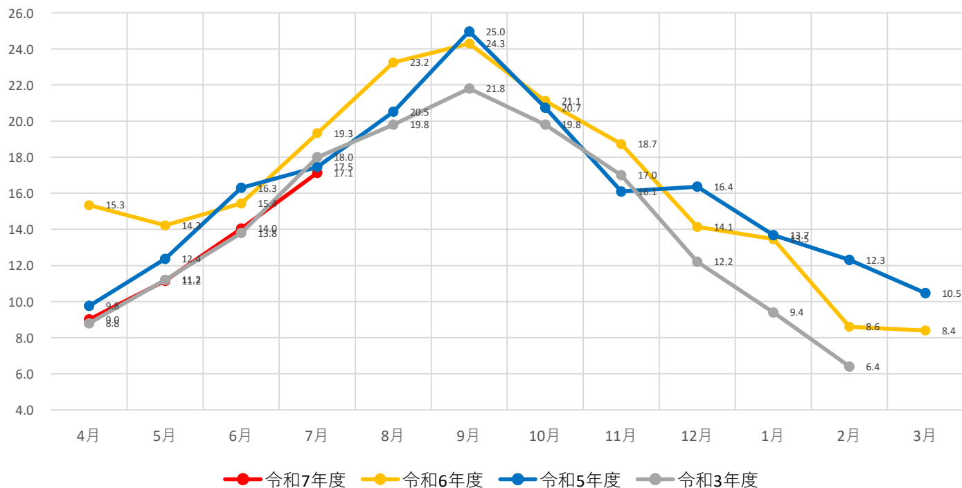
広田湾漁場水質調査 海水温各年度比較（要谷沖）
