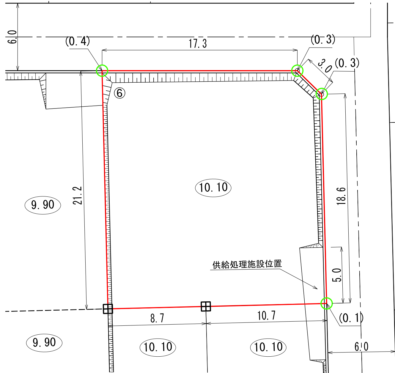
平面図 S=1:200(A3)
