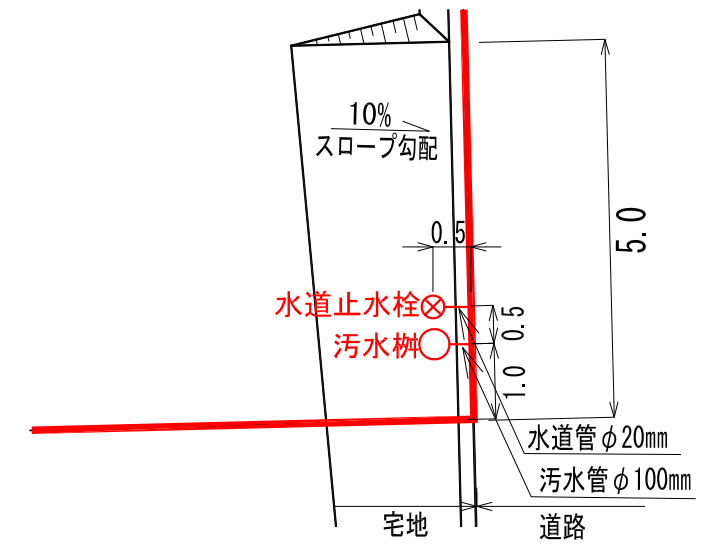
供給処理施設引込み位置図 S=1:100(A3)
