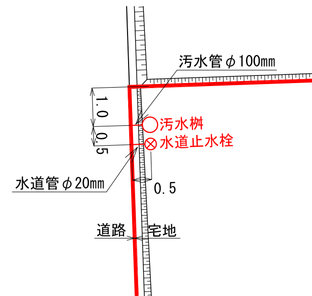
供給処理施設引込み位置図 S=1:100(A3)
