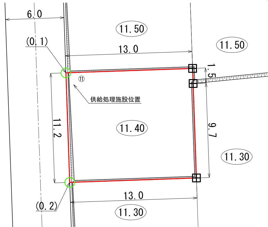
平面図 S=1:200(A3)
