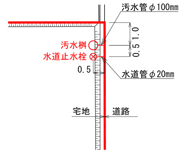
供給処理施設引込み位置図 S=1:100(A3)
