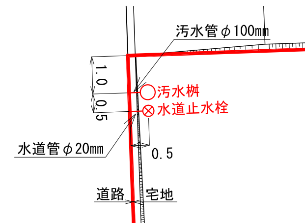
供給処理施設引込み位置図 S=1:100(A3)
