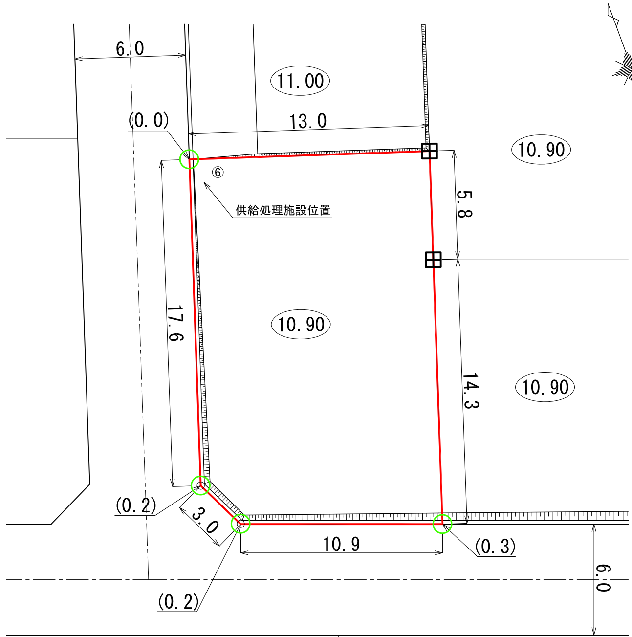
平面図 S=1:200(A3)
