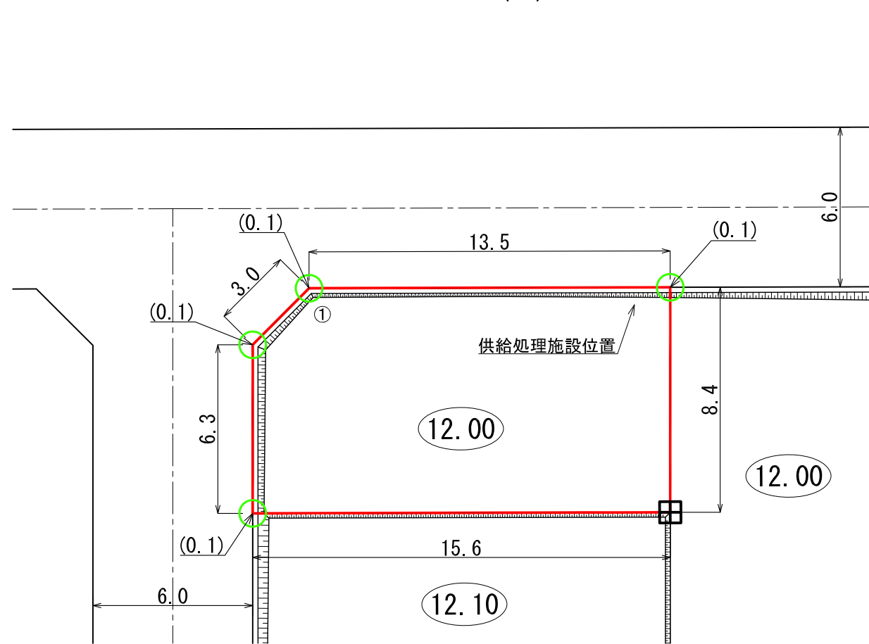
平面図 S=1:200(A3)
