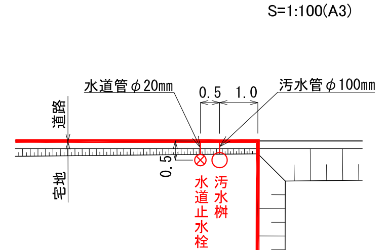
供給処理施設引込み位置図 S=1:100(A3)
