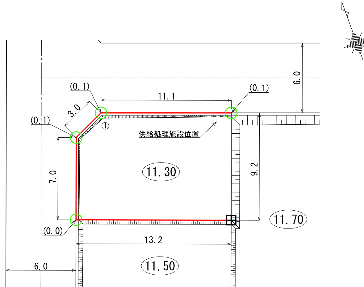
平面図 S=1:200(A3)
