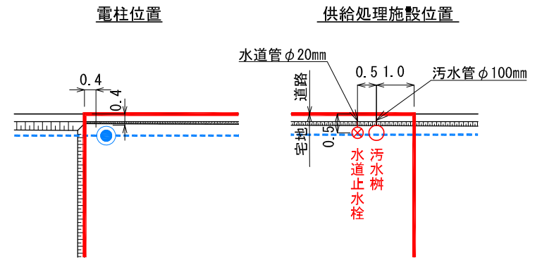
供給処理施設、電柱位置図 S=1:100(A3)
