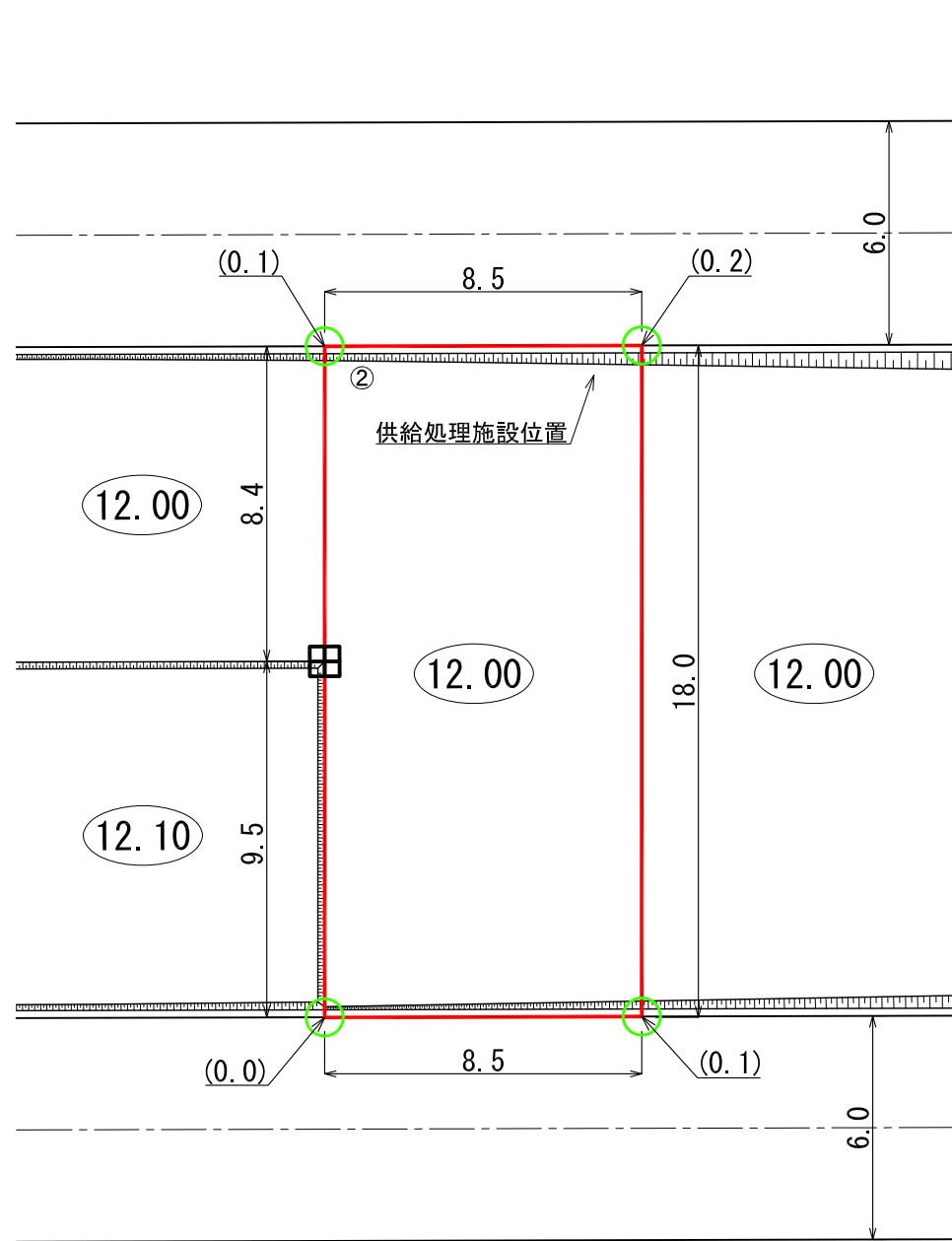
平面図 S=1:200(A3)
