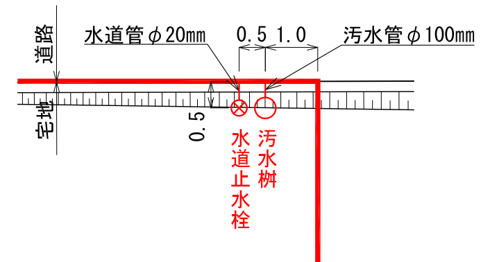
供給処理施設引込み位置図 S=1:100(A3)
