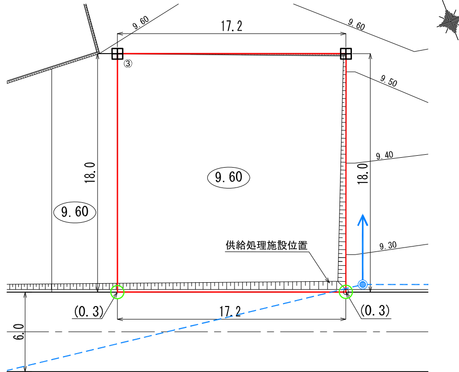
平面图
