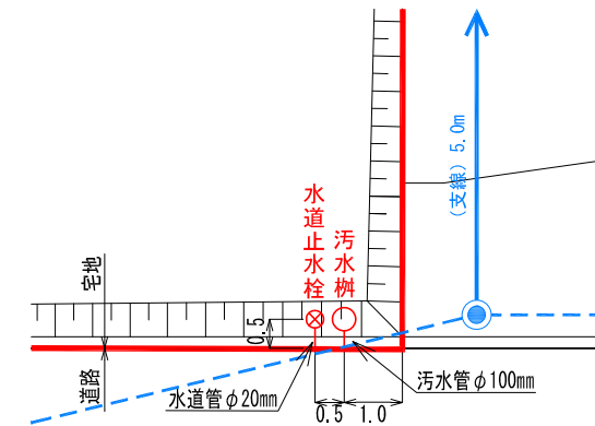
供給処理施設引込み位置図
