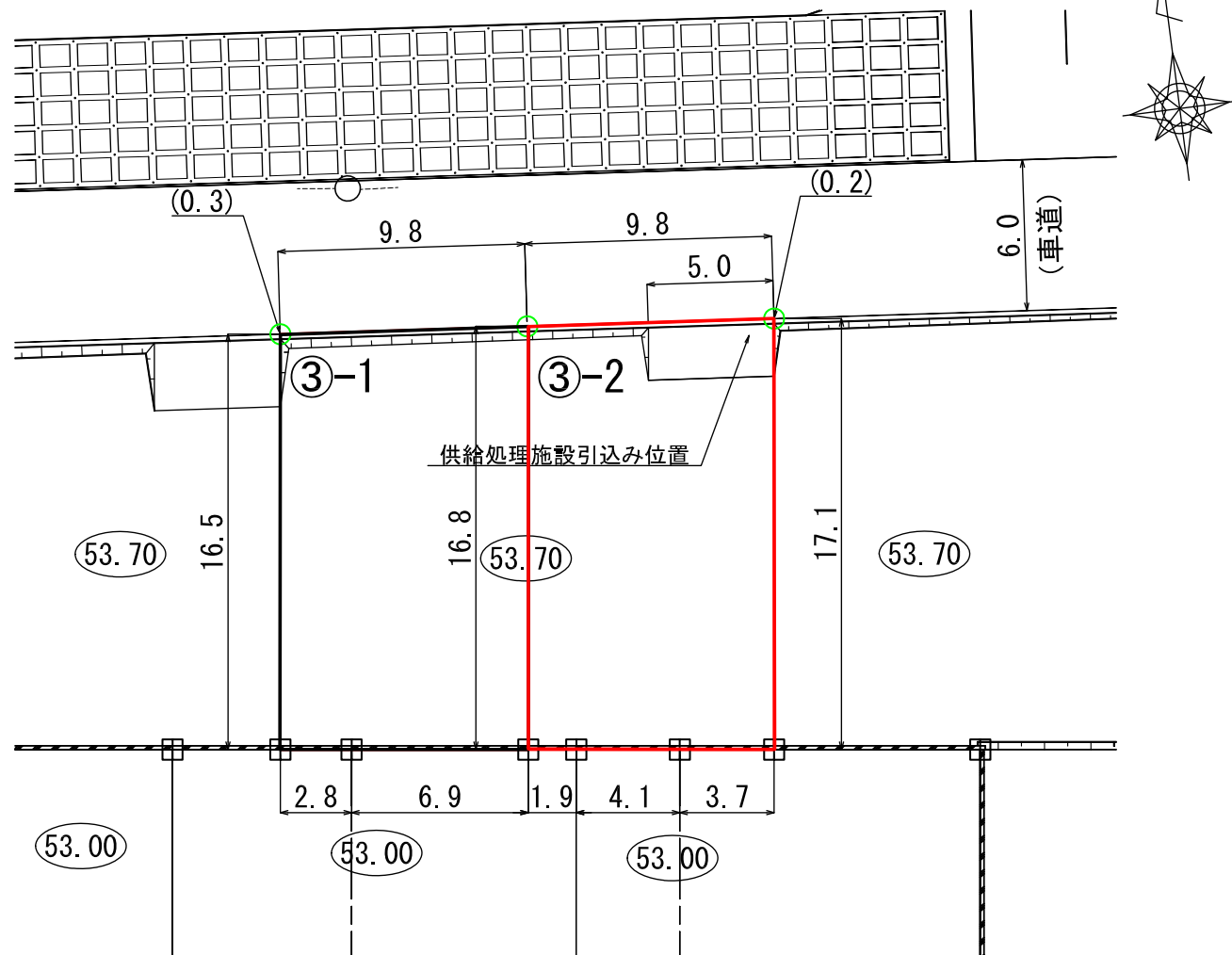
平面図 S:1:200
