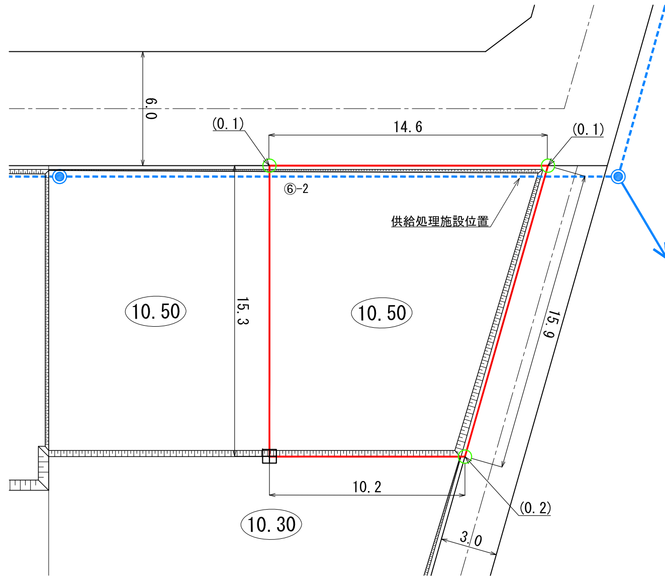
平面図 S=1:200(A3)
