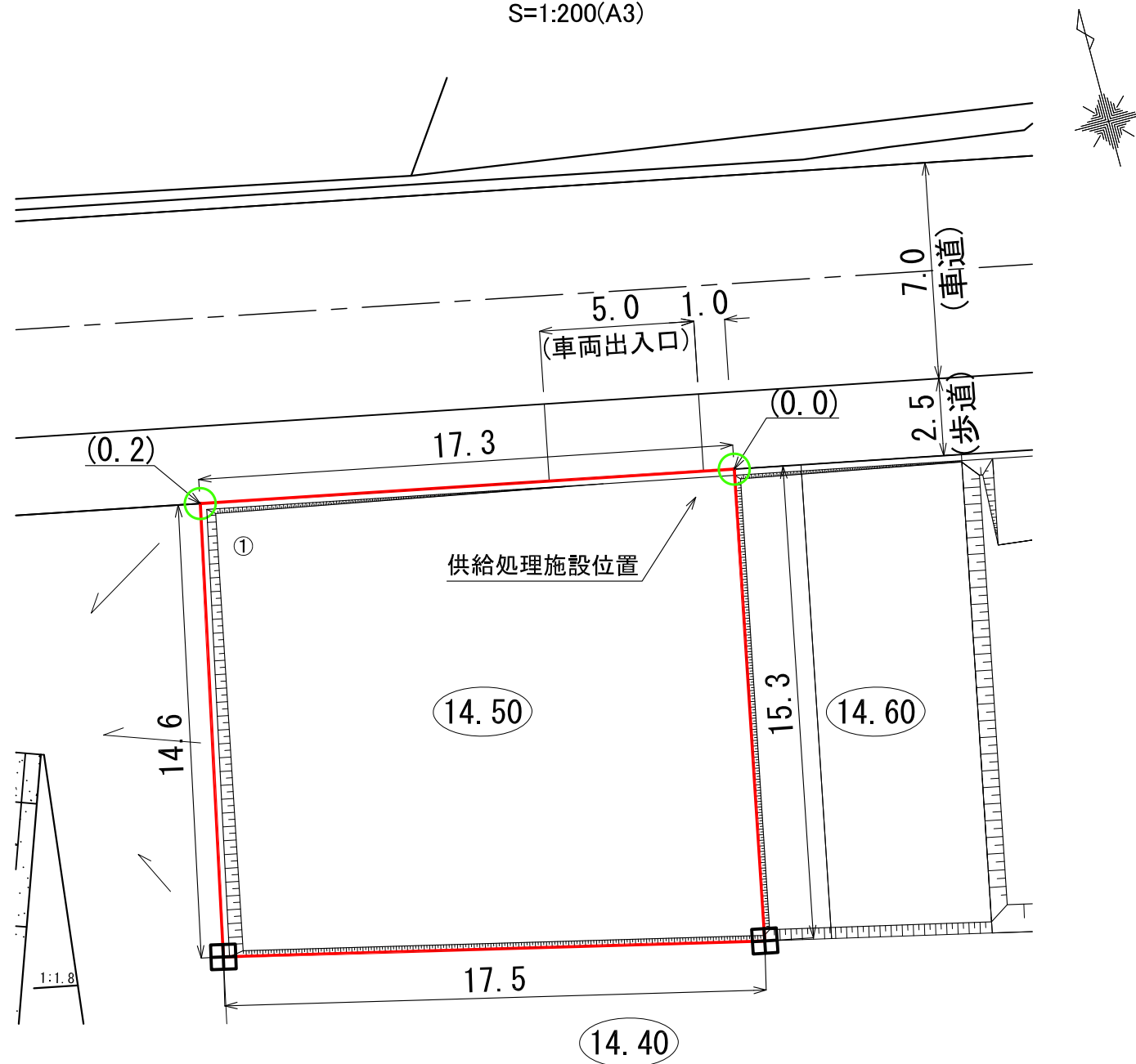
平面図 S=1:200(A3)
