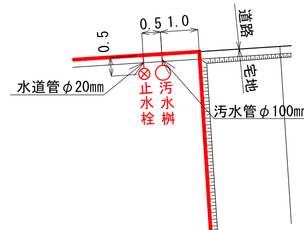
供給処理施設引込み位置図 S=1:100(A3)
