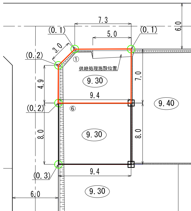
平面図 S=1:200(A3)
