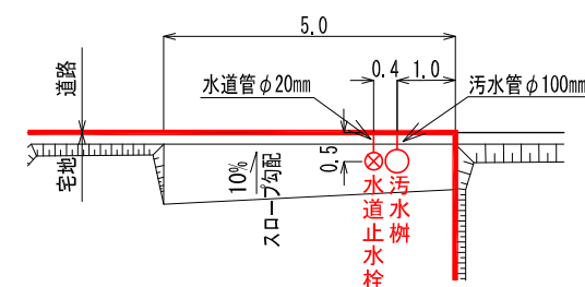
供給処理施設引込み位置図 S=1:100(A3)
