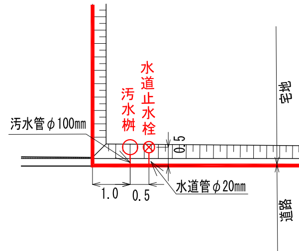
S=1:100(A3)
