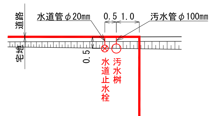
供給処理施設引込み位置図 S=1:100(A3)
