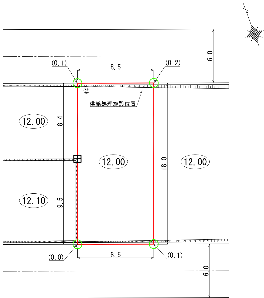
平面図 S=1:200(A3)
